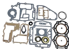
Tohatsu Gasket Set M35C, M40C 2 Cyl Replaces 361-87121-5M, 361-87121-3, 361-87121-1 Part No: 361-87121-5
